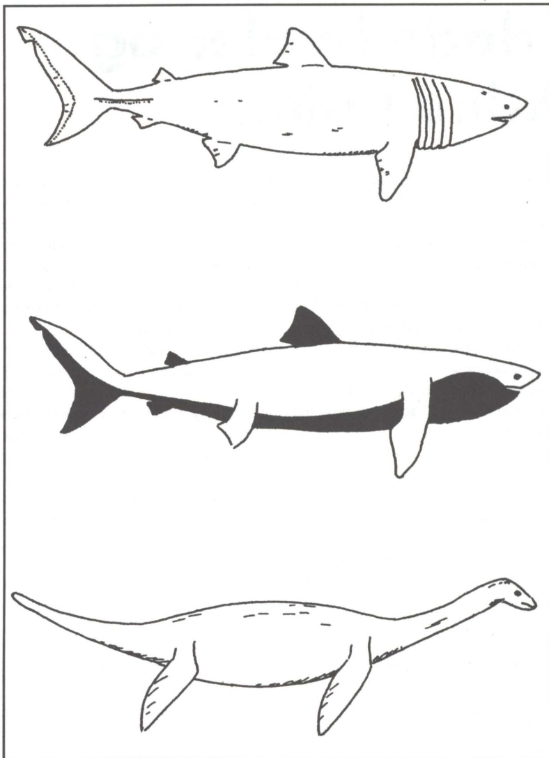
Lars Thomas har på disse tegninger vist, hvorledes en brugdehaj (øverst) ved forrådnelse kan komme til at ligne en svaneøgler (nederst). De sorte områder på den midterste tegning angiver de dele, der falder af ved forrådnelse.
